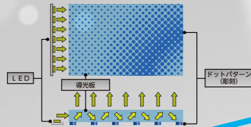
パターン彫刻 (レーザー導光板)
